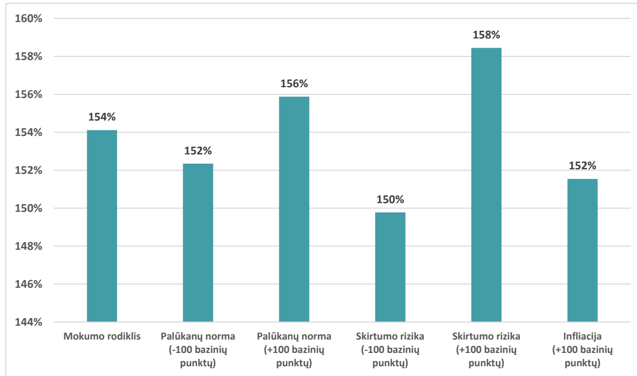
6 pav. Jautrumo analizės poveikis mokumo koeficientui
