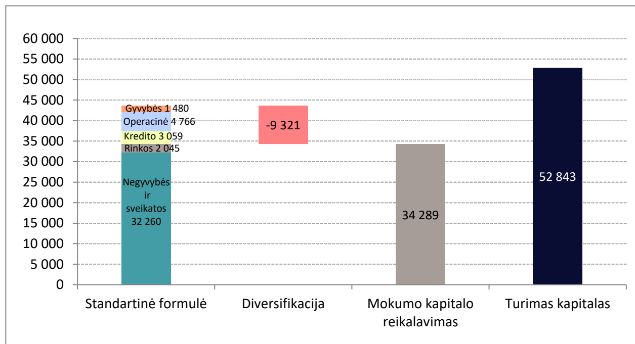
7 pav. ADB „Gjensidige“ kapitalo reikalavimas, apskaičiuotas pagal standartinę formulę
